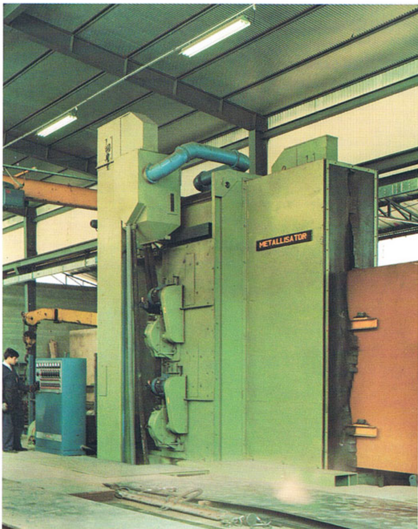
GRANIGLIATRICI VERTICALI PER LAMIERE VERTICAL SHOTBLAST UNITS FOR STEEL PLATES GRENAILLEUSES VERTICALES POUR TOLES
