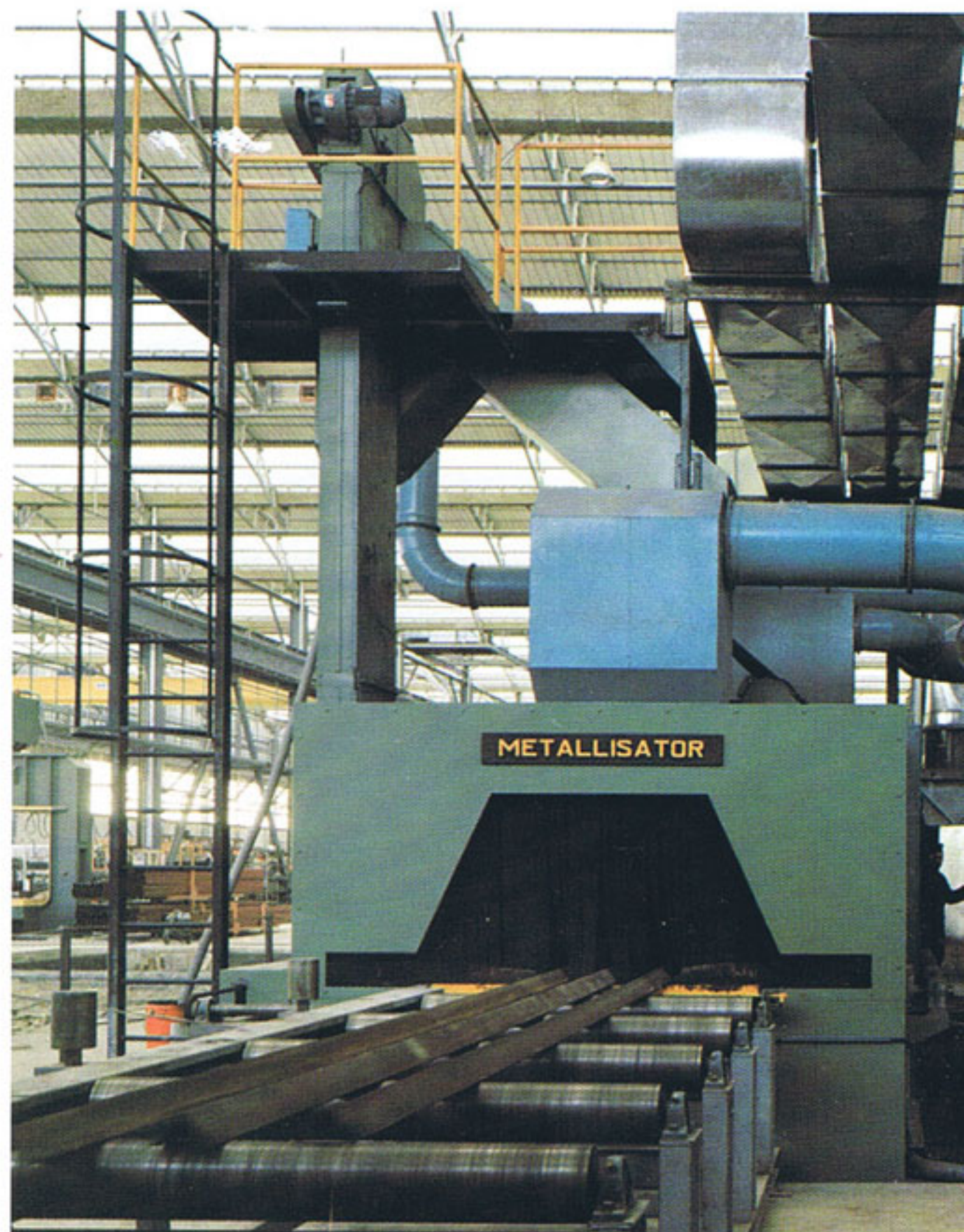
GRANIGLIATRICI ORIZZONTALI PER LAMIERE E PROFILATI HORIZONTAL SHOTBLAST UNITS FOR STEEL PLATES AND PROFILES GRENAILLEUSES HORIZONTALI POUR TOLES ET PROFILES
