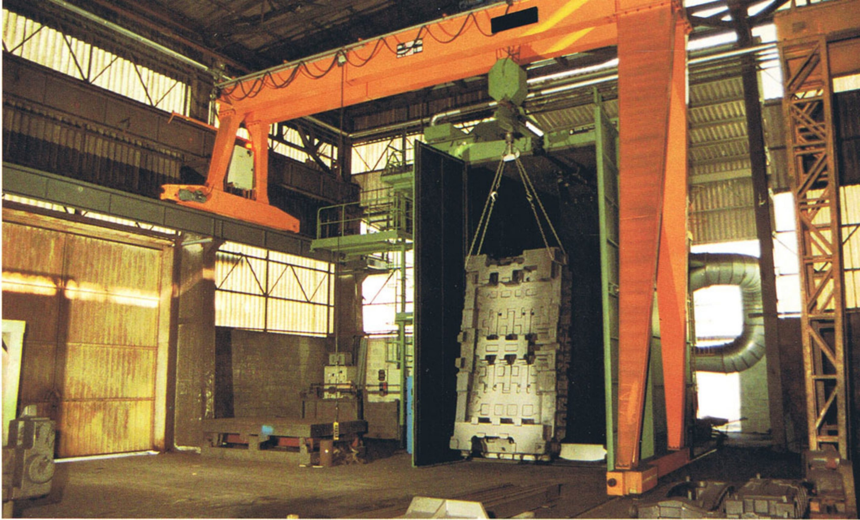
STERROGRANIGLIATRICI A CARROPONTE RADIOCOMANDATO. PORTATA 15 ÷ 40 TON DESANDING SHOTBLAST UNITS WITH RADIO CONTROLLED CRANE. CAPACITY 15 ÷ 40 TONS INSTALLATIONS DE DECOCHAGE ET GRENAILLAGE AVEC PONT ROULANT RADIOCOMMANDE. CAPACITE 15 ÷ 40 TONS
